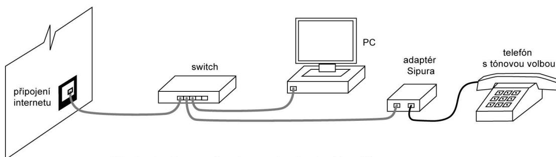
Obrázek: Doporučené zapojení adaptéru Sipura
