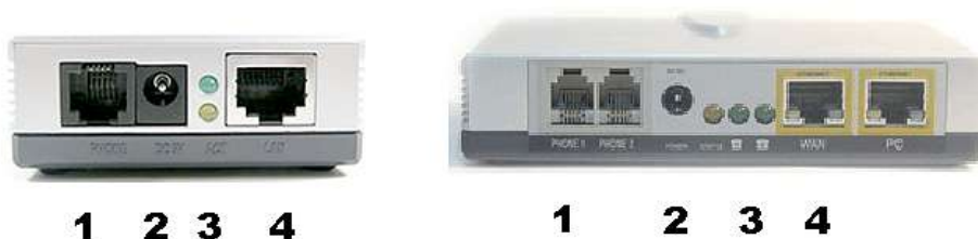
Obrázek . 1 - zadní strana adaptéru SPA -1001 a 2100 - (zleva) analogové výstupy na telefon(1); konektor napájení 5V(2); stavové diody)3); ethernetové konektory LAN/WAN a PC (4)
